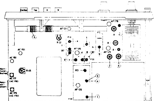
Abgleich-Lageplan
